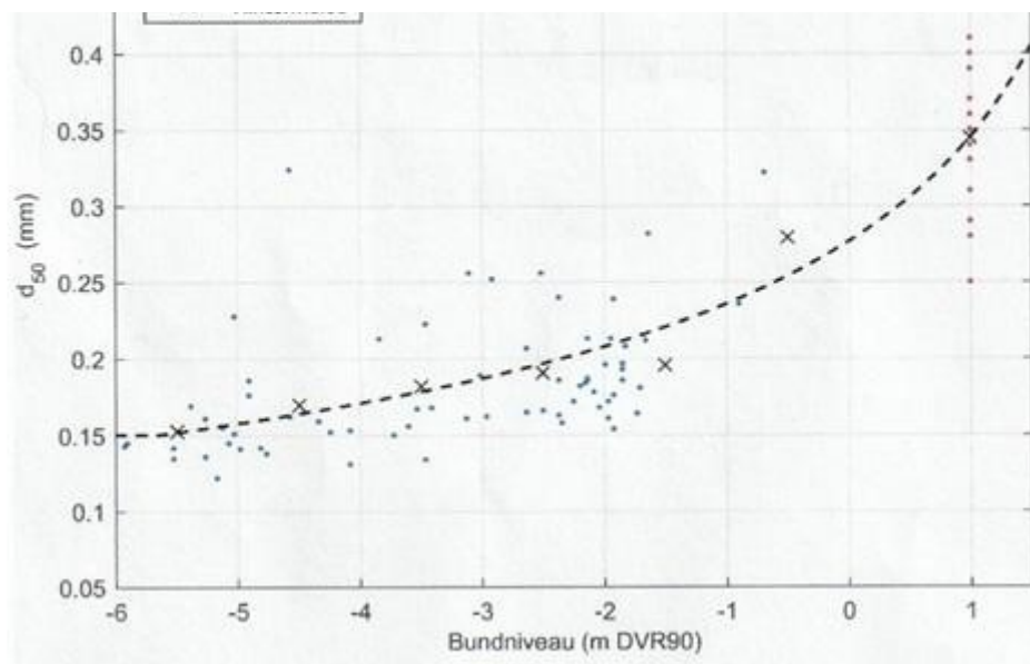
Figur 5. Sammenhæng mellem sedimentets middelhørnstørrelse og bundniveau i forhold til havoverfladen. Illustration: Dansk Hydraulisk Institut. Illustration: Dansk Hydraulisk Institut.
